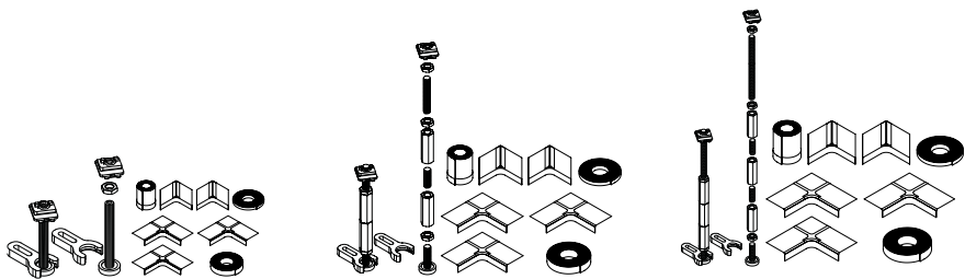
Hauteur de montage 4,5 - 11 cm Hauteur de montage 10 - 20 cm Hauteur de montage 19 - 33 cm
