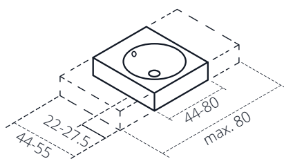
Lavabo in mezzo
