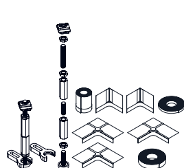
Altezza di montaggio 10 - 20 cm
